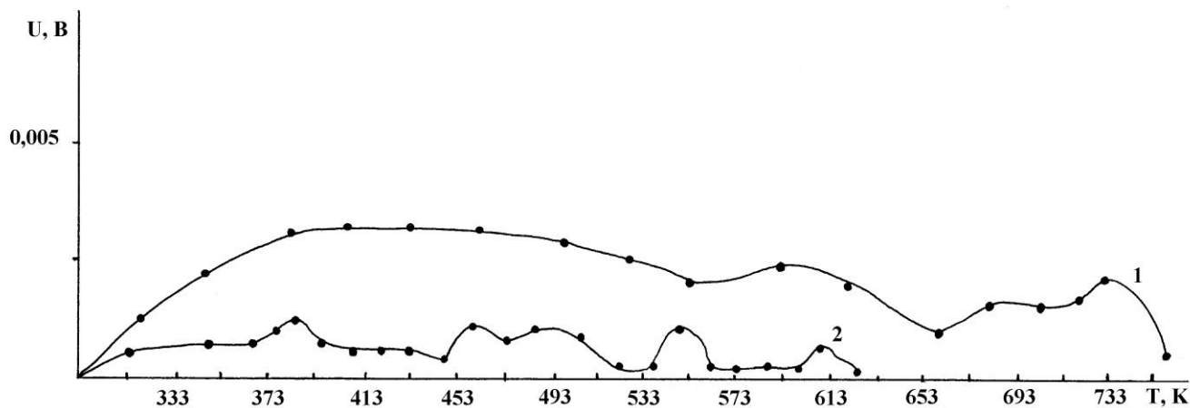
Рис. 5. Термодесорбционные кривые выделения кислорода (32 масса) с поверхности CdTe – 1 и КРТ-ИР - 2 при P_{\text{нач}} = 10 Па , t_{\text{адс}} = 60 мин
