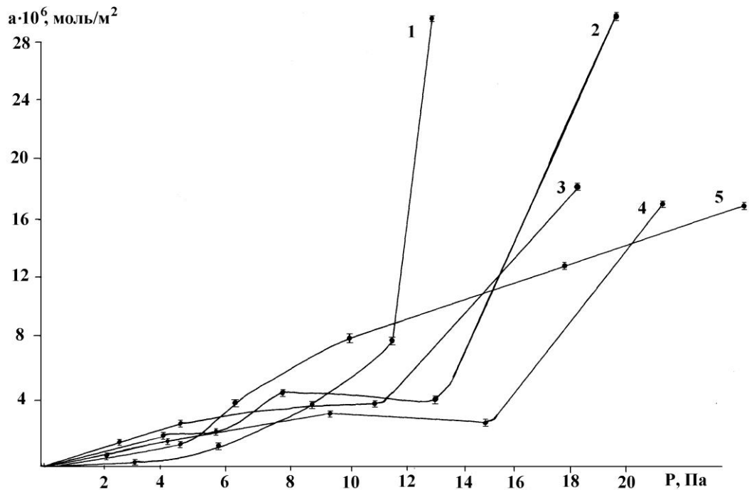
Рис. 1. Кривые изменения величины адсорбции кислорода от давления на монокристаллах КРТ-ИР ( S_{\text{удел. геом}} = 39,2 \text{ м}^2/\text{кг} ): 1 - 323 К, 2 - 275 К, 3 - 373 К, 4 – 253, 5 – 294 К
